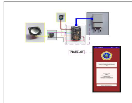
Gambar 7. Rangkaian Sistem
