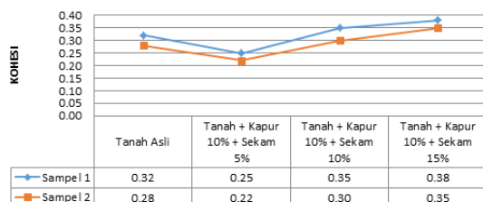
Gambar 12. Grafik Nilai Kohesi Pengujian Kuat Geser Pemeraman 7 Hari
