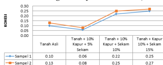
Gambar 8. Grafik Nilai Kohesi Pengujian Kuat Geser Pemeraman 0 Hari
