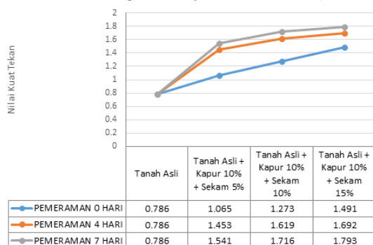
Gambar 6. Hasil Pengujian Kuat Tekan Bebas Pada Sampel 1
