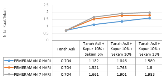
Gambar 7. Hasil Pengujian Kuat Tekan Bebas Pada Sampel 1
