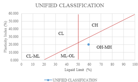
Gambar 5. Klasifikasi Tanah menurut USCS pada sampel 2
