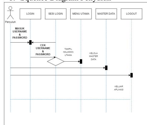
Gambar 3. Sequence Diagram Penyuluh
