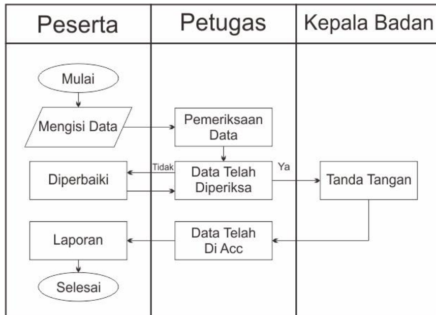
Gambar 1 Flow Map Sistem yang sedang berjalan
