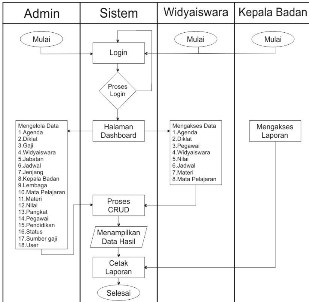
Gambar 2 Flow Map Sistem yang diusulkan
