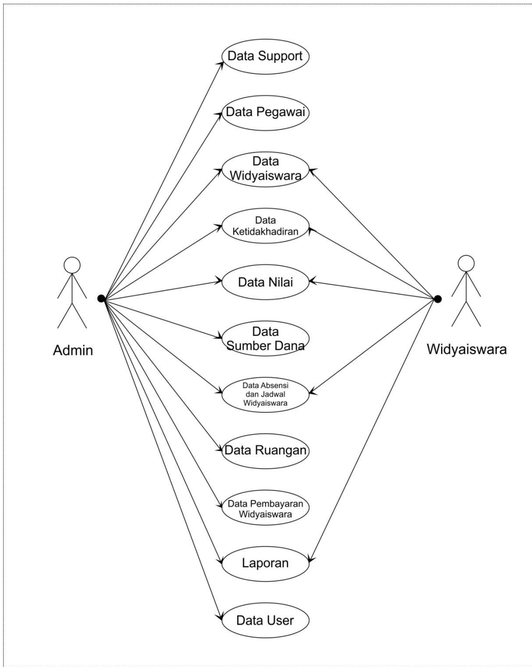
Gambar 3 Use Case Diagram sistem yang diusulkan
