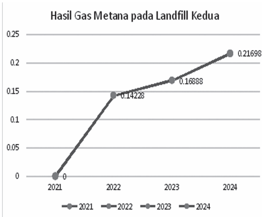
Gambar 4.13 Grafik Hasil Gas Metana Landfill Kedua Metode IPCC
