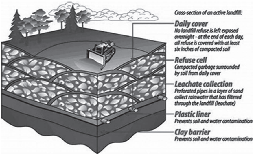
Gambar 4.7 Denah Potongan Landfill beserta Tingginya
