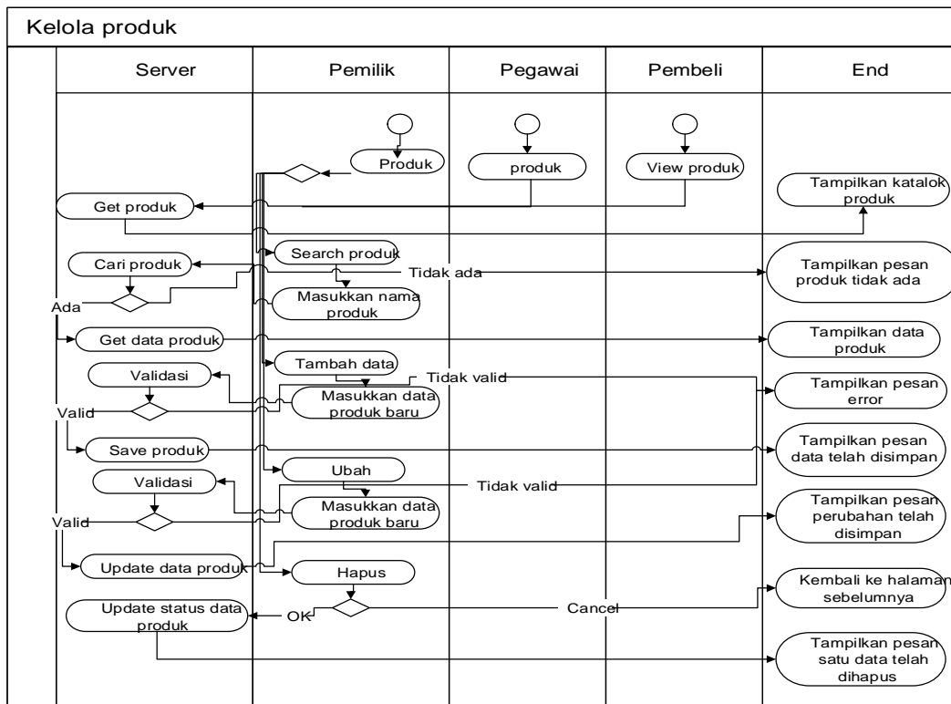
Gambar 1. 3 Activity Diagram Kelola Produk
