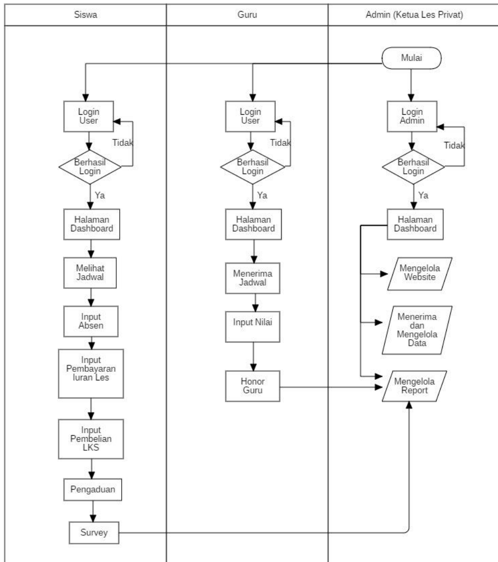
Gambar 1. 2 Sistem yang di usulkan
