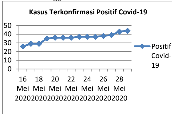
Gambar 2. Pertumbuhan Covid-19 Pertanggal 16 Mei-29 Mei 2020.
