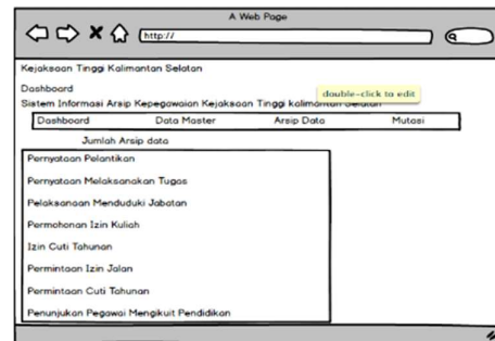
Gambar 8 Rancangan Beranda Admin
