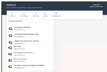
Gambar 13 Tampilan Beranda
