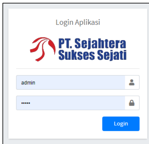
Gambar 1. 9 Halaman Login
