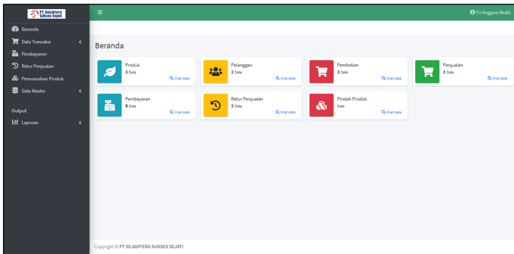
Gambar 1. 10 Halaman Beranda
