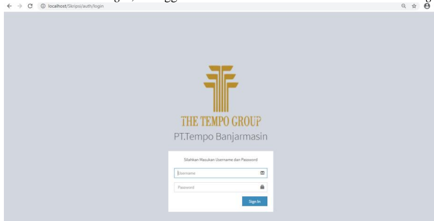
Gambar 4. 1 Menu Login
