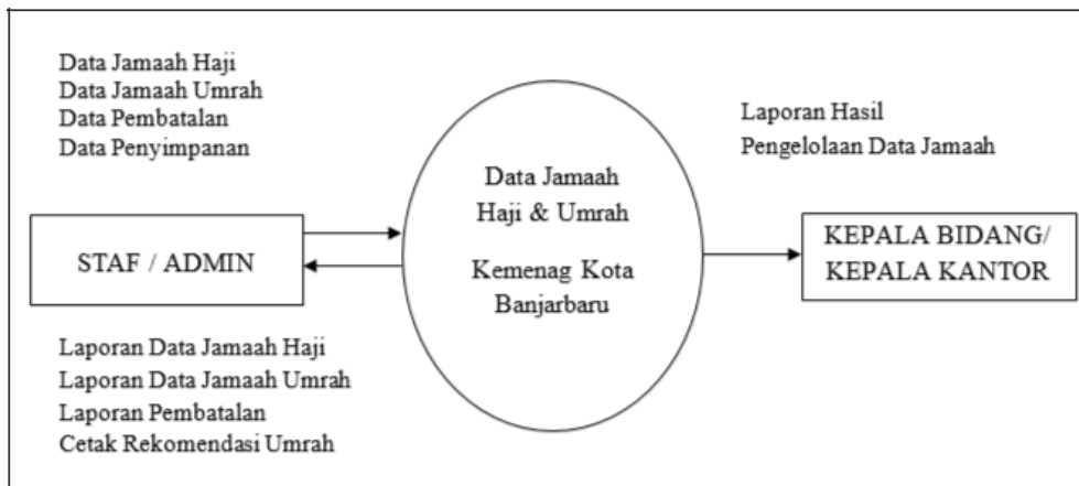
Gambar 2. Diagram Konteks
