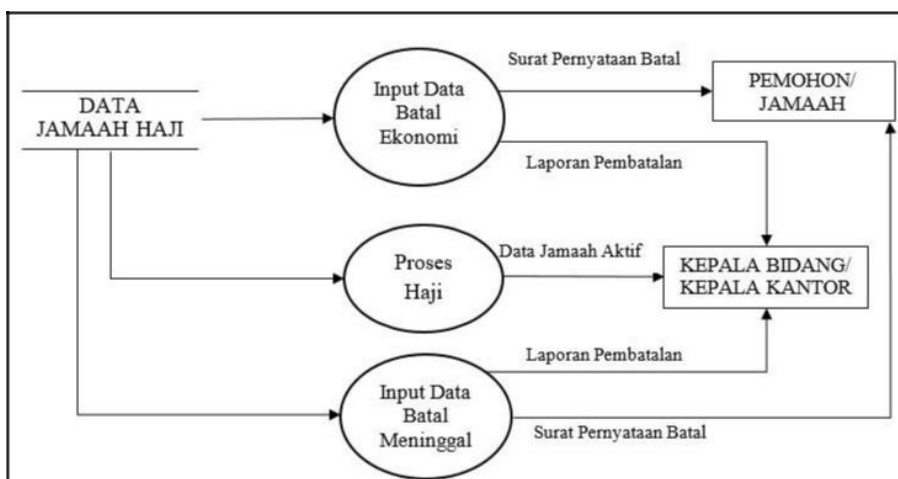
Gambar 4. DFD Level 2
