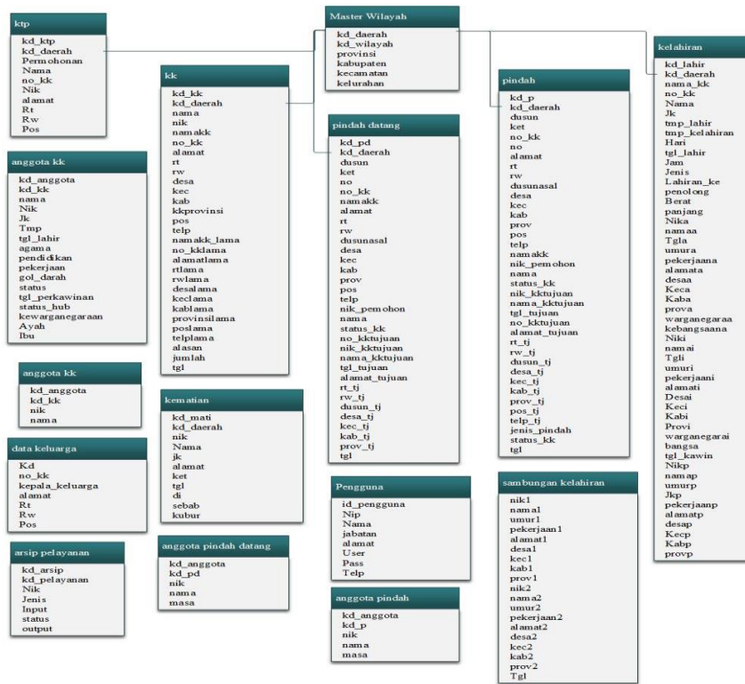
Gambar 3. 7 Relasi Tabel 1
